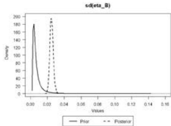
(b) Parameter sd(\eta^B)
