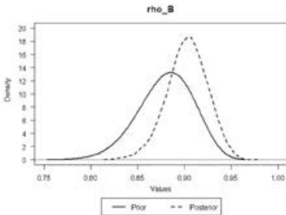
(a) Parameter \rho^B
